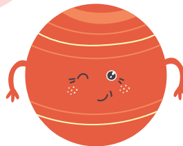
Jupiter
