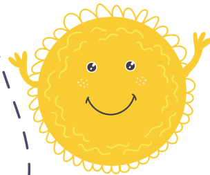
Sun
